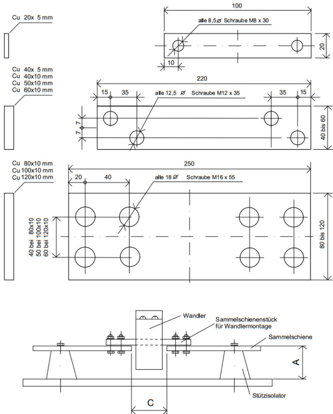
Abbildung 11: Details zu demontierbaren Sammelschienenstücken
